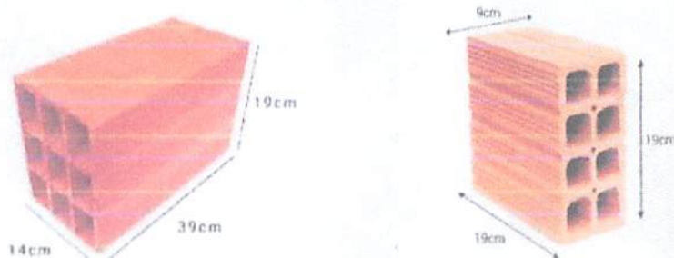
Imagem 02: Ilustração do bloco cerâmico que está sendo utilizado em obra (9x19x19) e do bloco cerâmico que está previsto em planilha (14x19x39).
