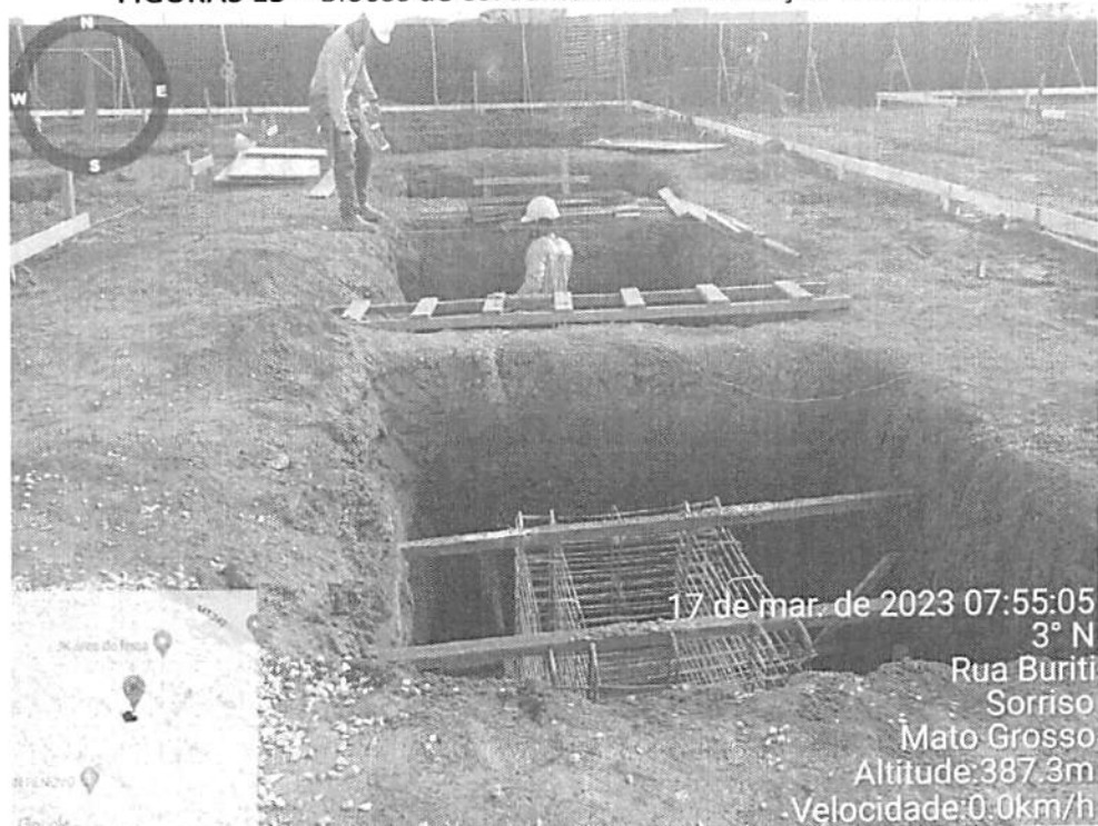
FIGURAS 13 – Blocos de coroamento com armação dos cálices
