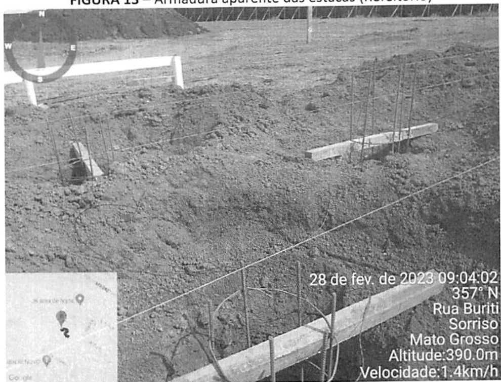
FIGURA 13 – Armadura aparente das estacas (Refeitório)
