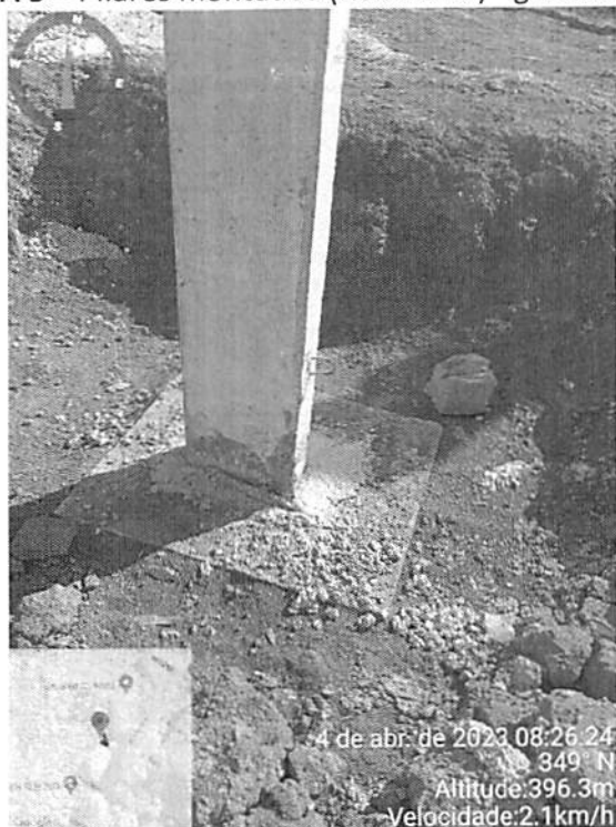
FIGURA 5 – Pilares montados (Refeitório) - grauteamento
