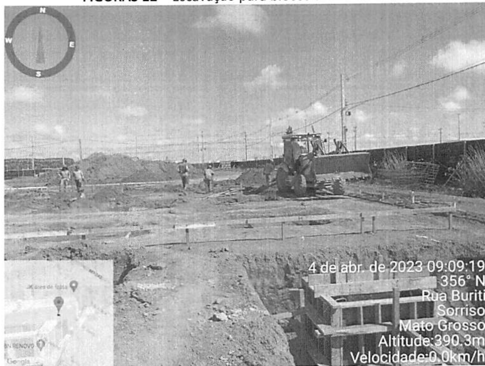
FIGURAS 12 – Escavação para blocos de coroamento
