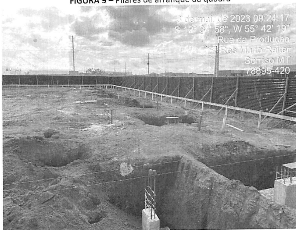
FIGURA 9 – Pilares de arranque da quadra
