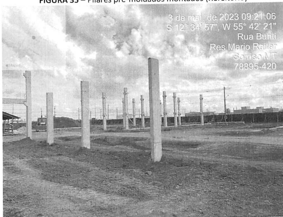
FIGURA 35 – Pilares pré-moldados montados (Refeitório)
