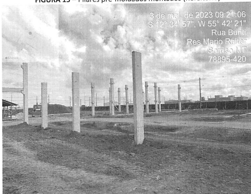
FIGURA 15 – Pilares pré-moldados montados (Refeitório)
