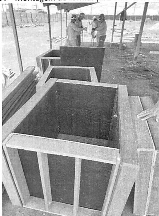
FIGURA 14 – Montagem de fôrmas para blocos de coroamento
