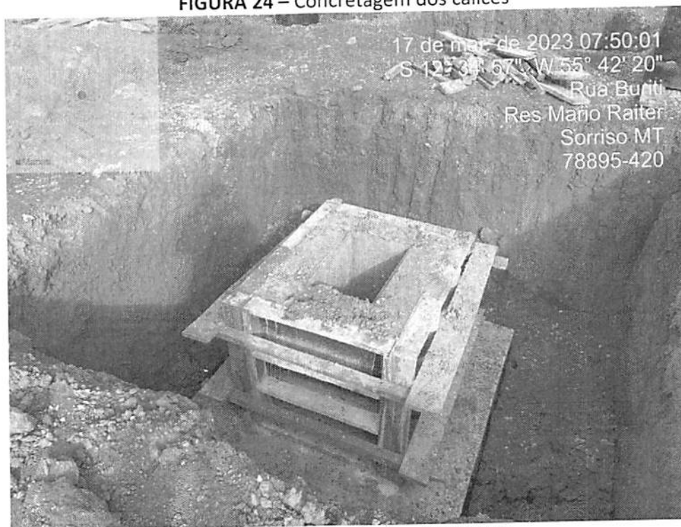
FIGURA 24 – Concretagem dos cálices
