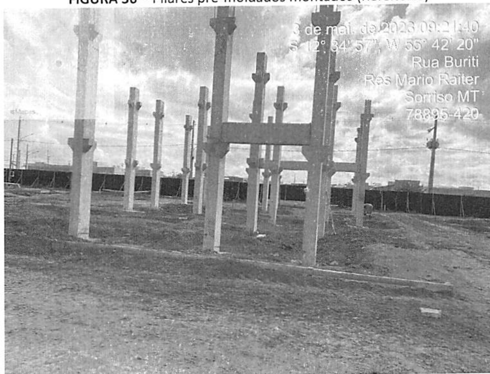
FIGURA 36 – Pilares pré-moldados montados (Refeitório)
