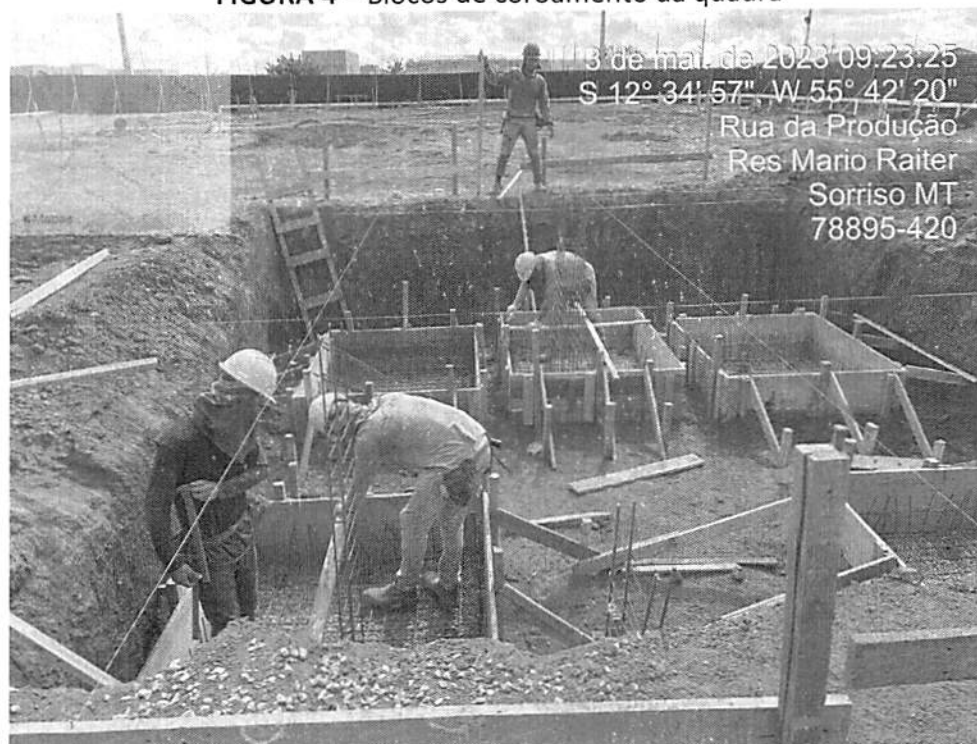
FIGURA 4 – Blocos de coroamento da quadra
