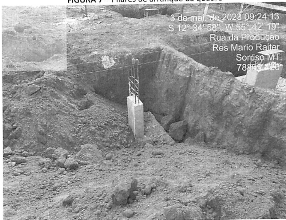
FIGURA 7 – Pilares de arranque da quadra
