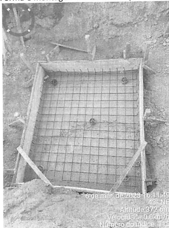
FIGURA 17 – Fôrma e montagem de armadura para blocos coroamento
