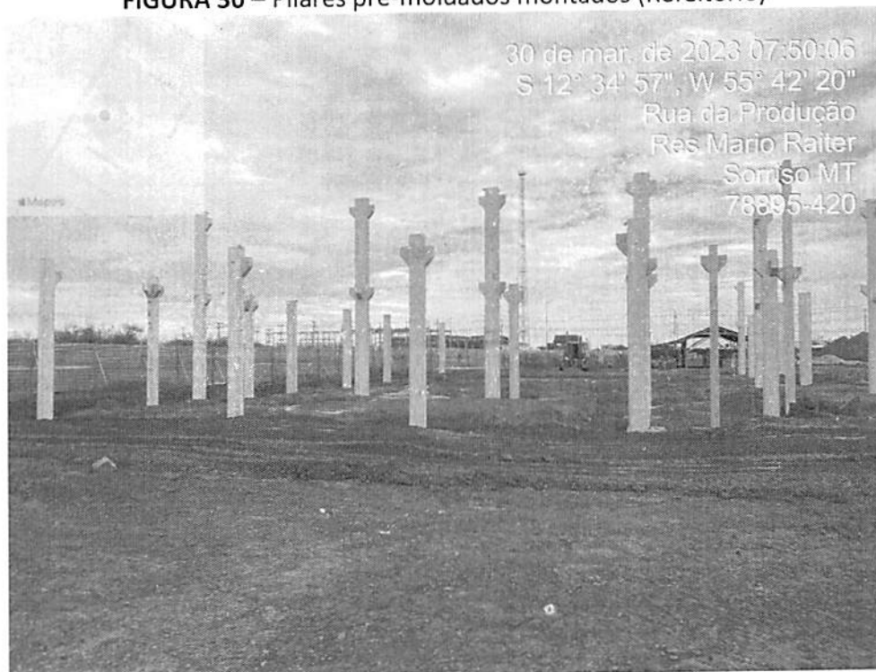
FIGURA 30 – Pilares pré-moldados montados (Refeitório)
