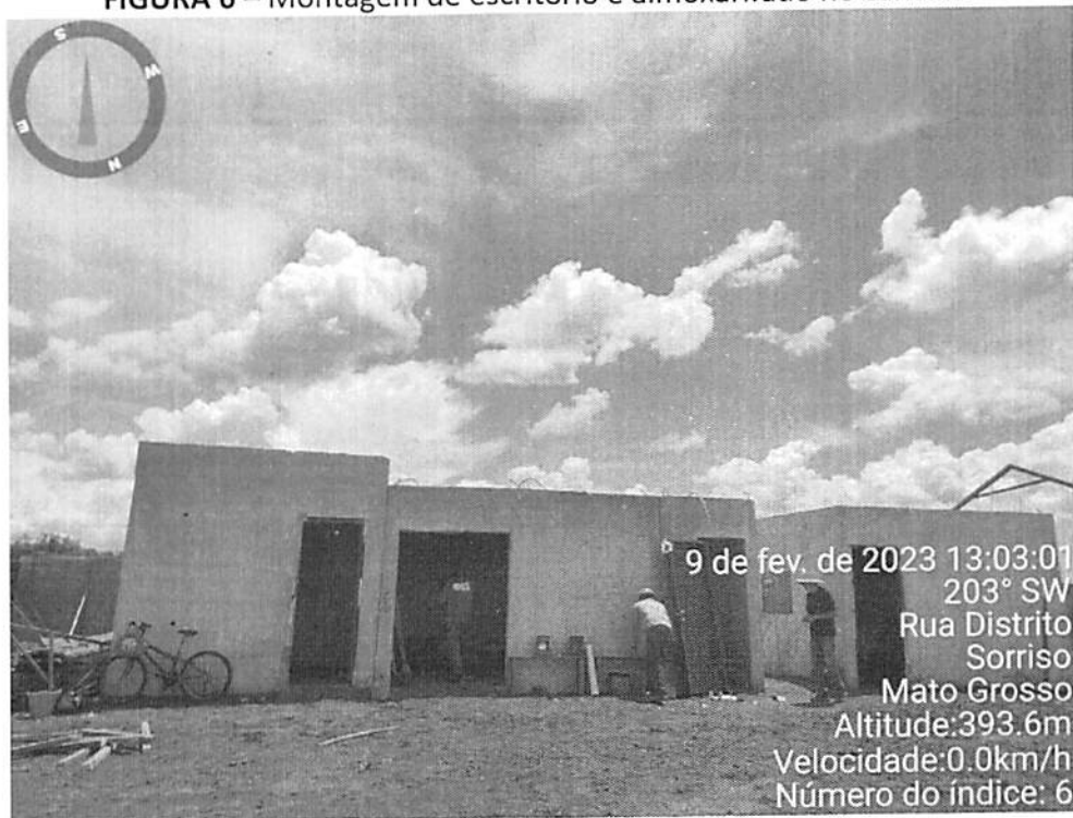
FIGURA 6 – Montagem de escritório e almoxarifado no canteiro
