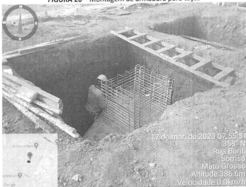
FIGURA 20 – Montagem de armadura para taças
