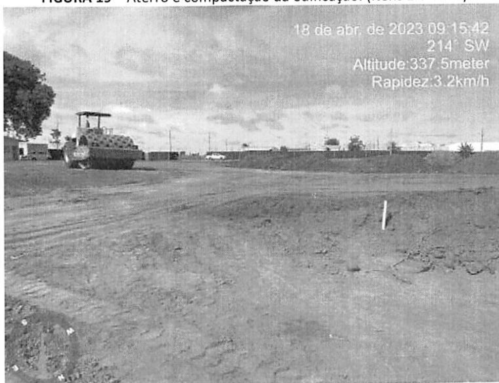
FIGURA 19 – Aterro e compactação da edificação. (Itens 2.3 e 2.4)
