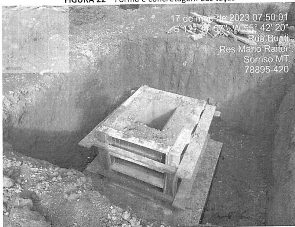
FIGURA 22 – Fôrma e concretagem das taças
