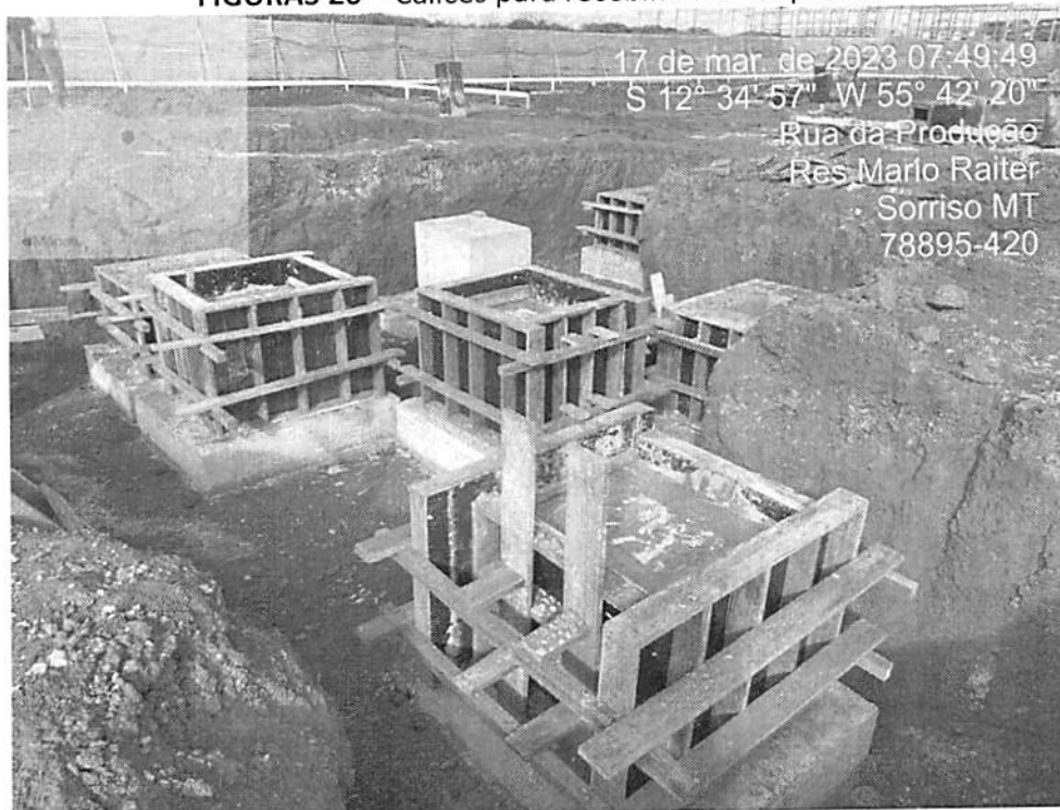
FIGURAS 26 – Cálices para recebimento de pilares
