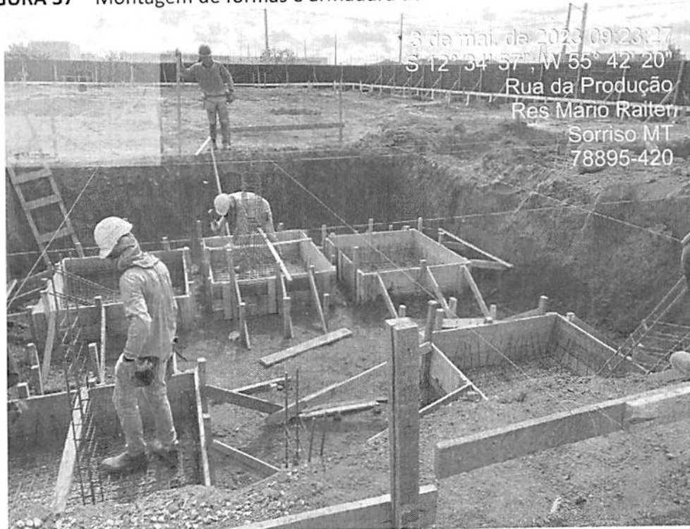
FIGURA 37 – Montagem de fôrmas e armadura dos blocos de coroamento (Quadra)
