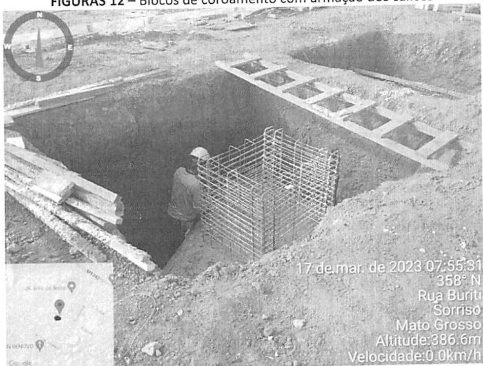
FIGURAS 12 – Blocos de coroamento com armação dos cálices
