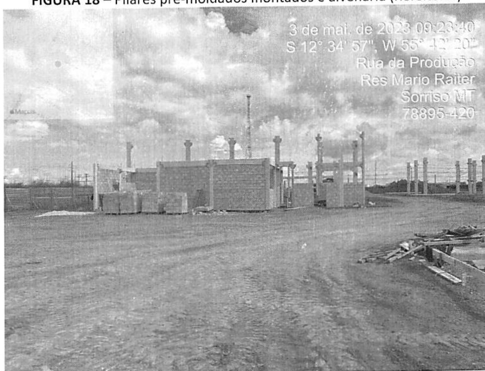
FIGURA 18 – Pilares pré-moldados montados e alvenaria (Refeitório)
