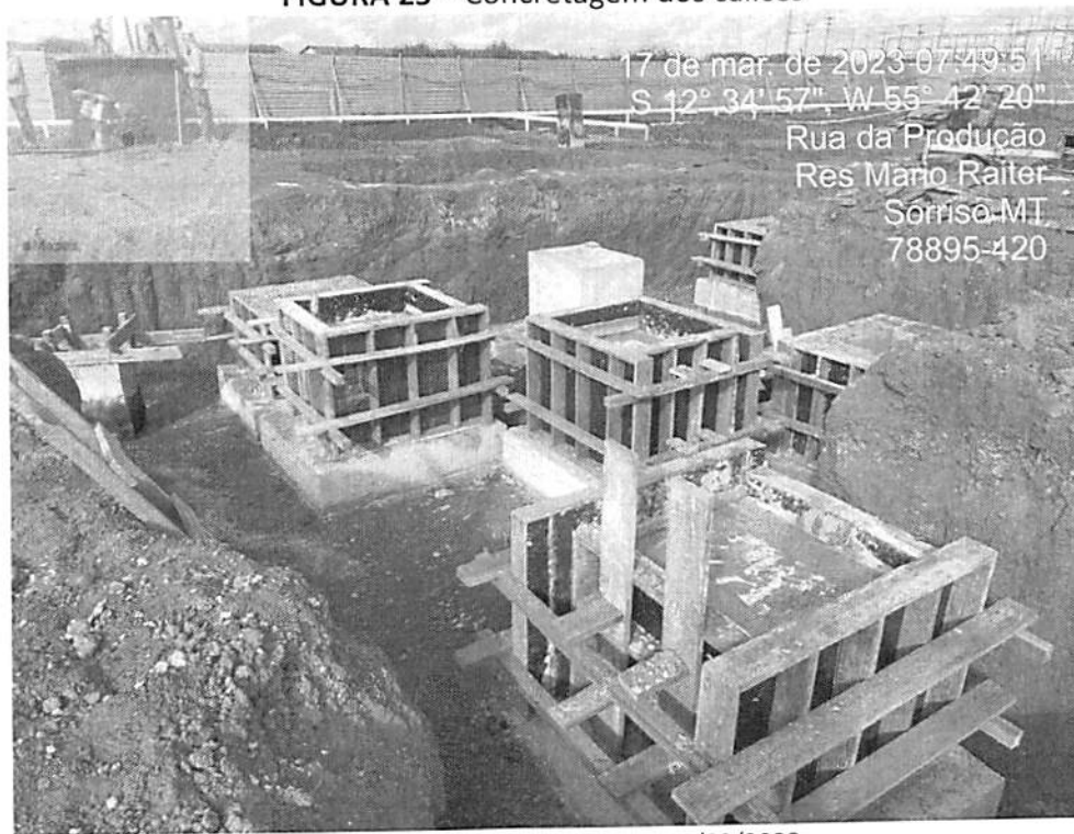
FIGURA 23 – Concretagem dos cálices
