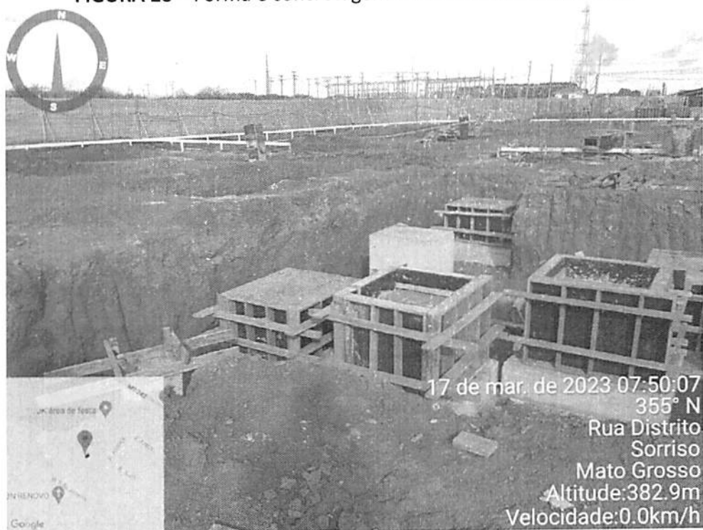
FIGURA 28 – Fôrma e concretagem dos blocos de coroamento
