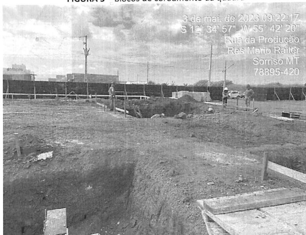
FIGURA 3 – Blocos de coroamento da quadra
