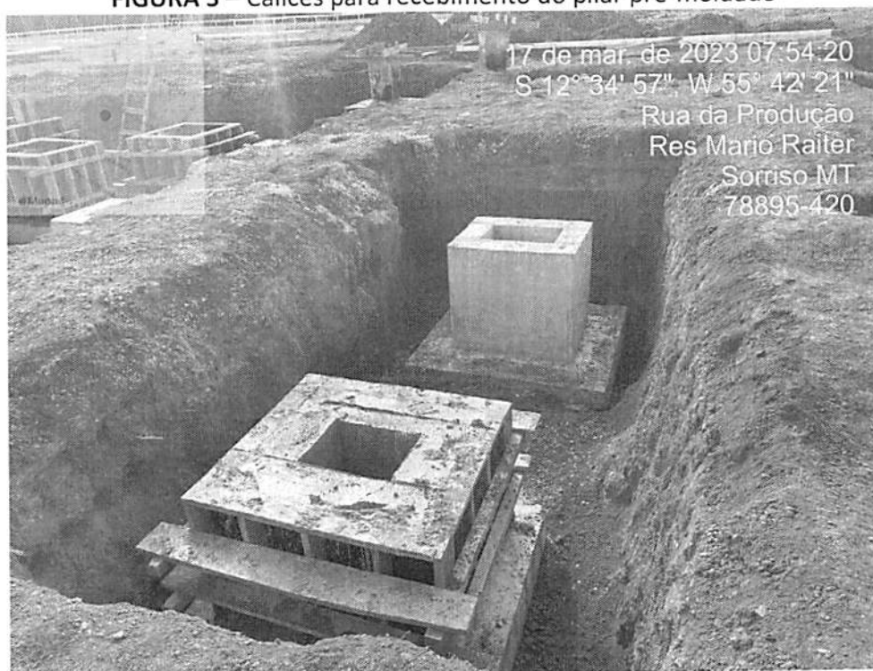
FIGURA 3 – Cálices para recebimento do pilar pré-moldado
