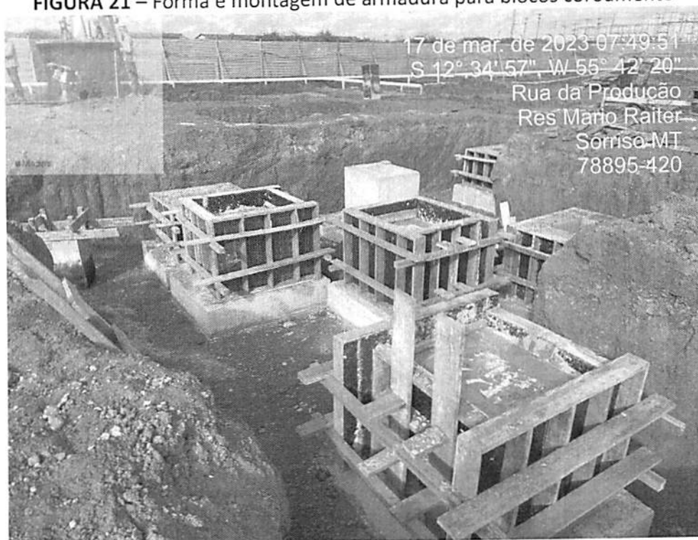
FIGURA 21 – Fôrma e montagem de armadura para blocos coroamento
