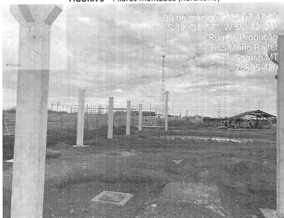
FIGURA 3 – Pilares montados (Refeitório)
