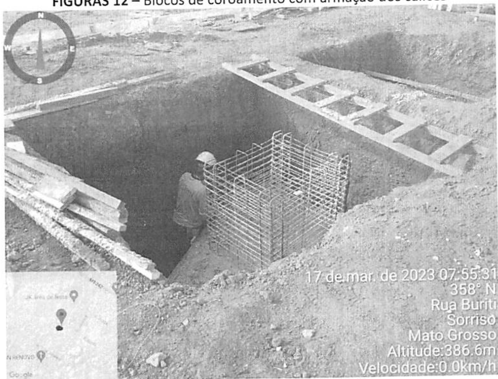
FIGURAS 12 – Blocos de coroamento com armação dos cálices
