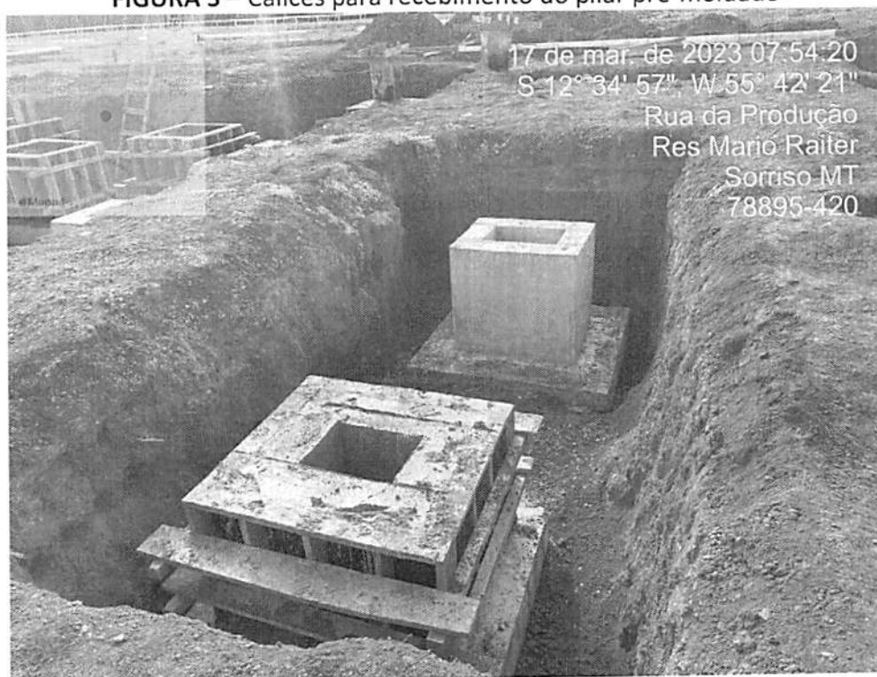
FIGURA 3 – Cálices para recebimento do pilar pré-moldado
