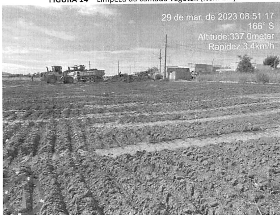
FIGURA 14 – Limpeza da camada vegetal. (Item 2.1)
