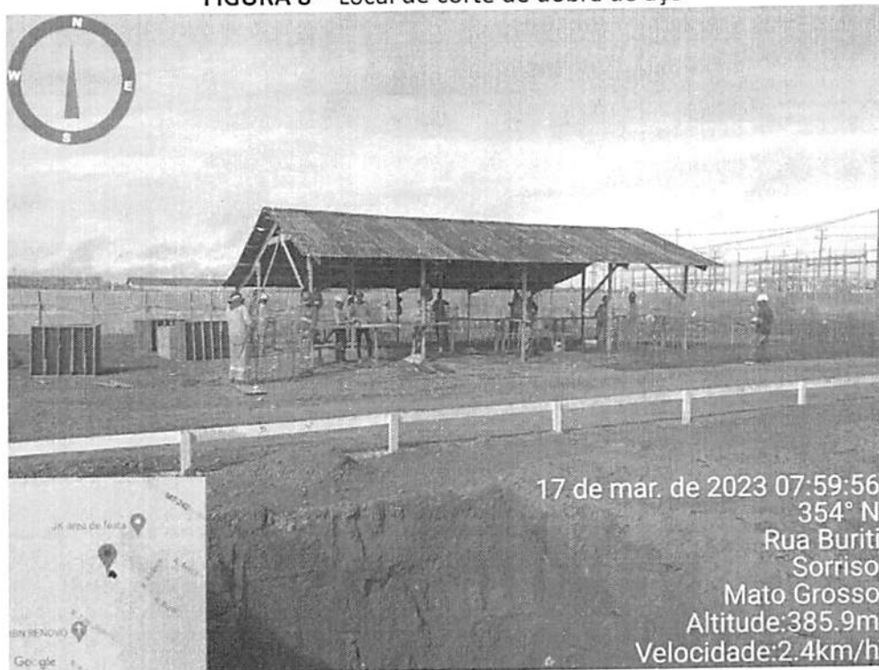
FIGURA 8 – Local de corte de dobra de aço
