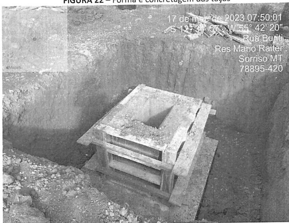
FIGURA 22 – Fôrma e concretagem das taças
