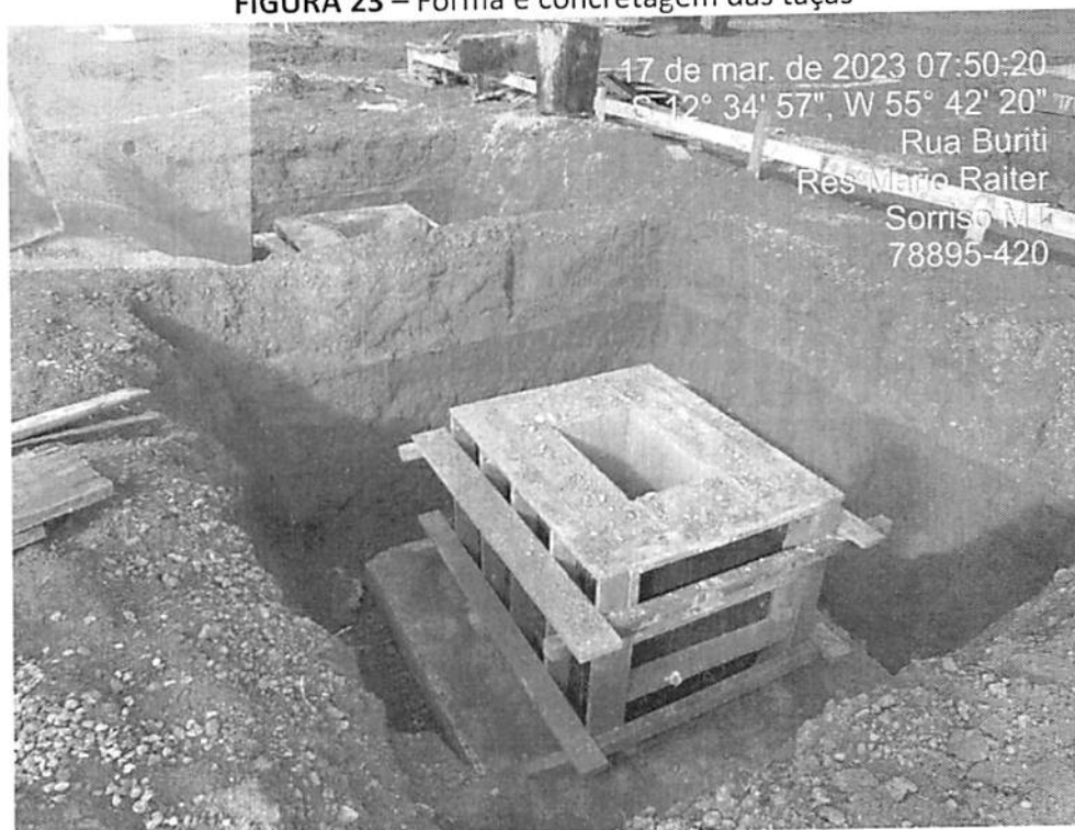
FIGURA 23 – Fôrma e concretagem das taças
