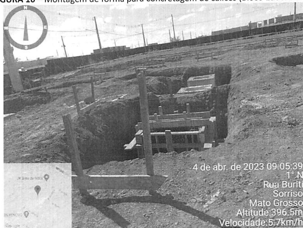
FIGURA 10 – Montagem de fôrma para concretagem de cálices (Bloco Educacional)
