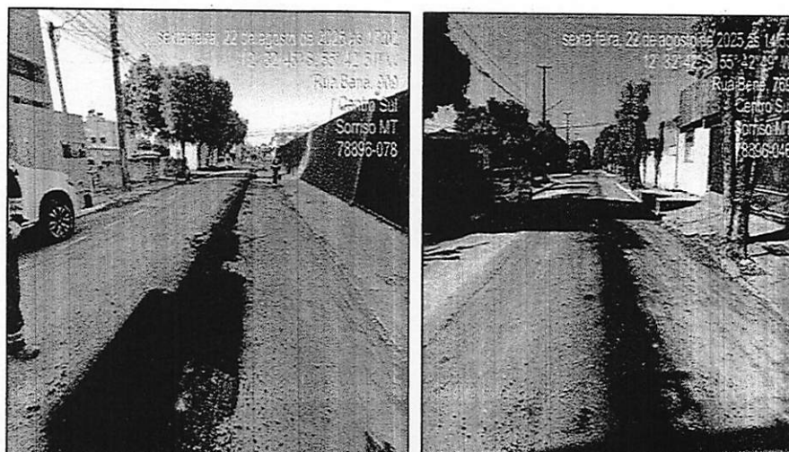
Figura 18. Recomposição da camada asfáltica
