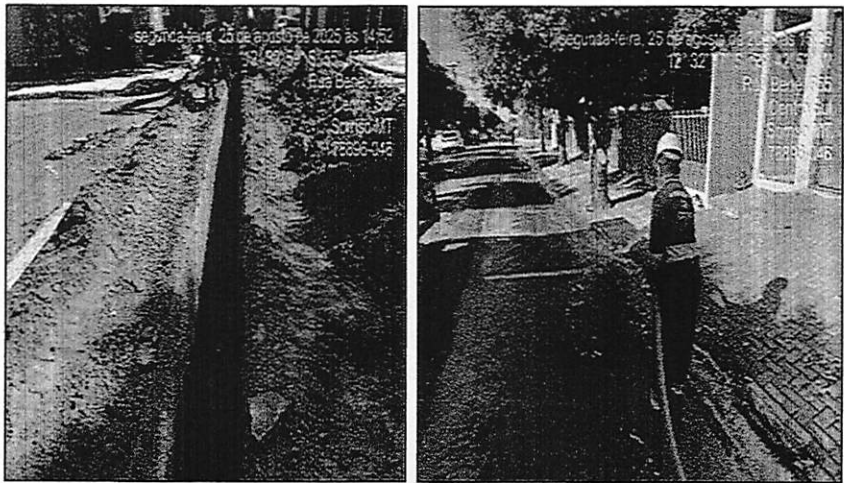
Figura 26. Assentamento de tubos e limpeza da área
