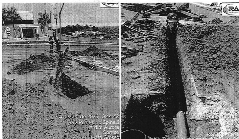
Figura 5. Escavação e assentamento de tubos, rede coletora.
