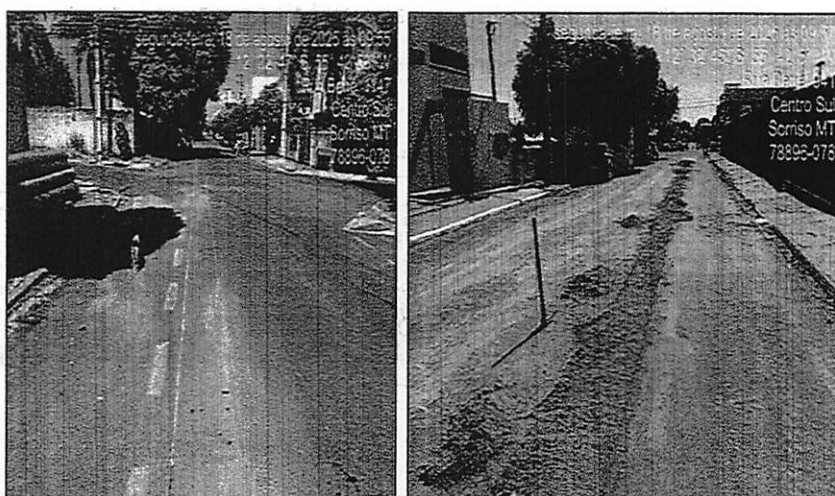
Figura 2. Implantação de rede de esgoto
