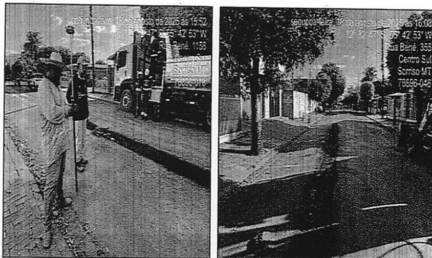
Figura 3. Levantamento topográfico e recomposição da vala
