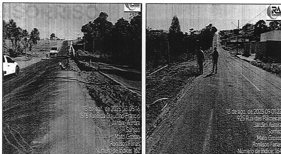
Figura 4. Assentamento de tubos e levantamento topográfico
