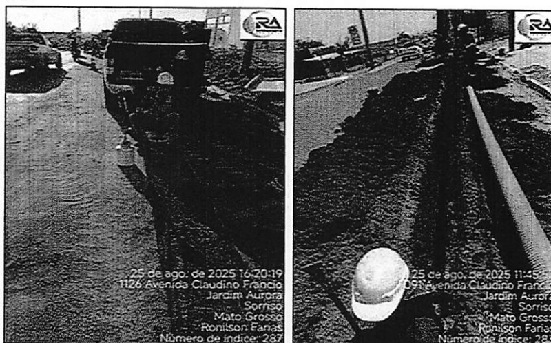
Figura 28. Análise da compactação do solo após instalação de tubo
