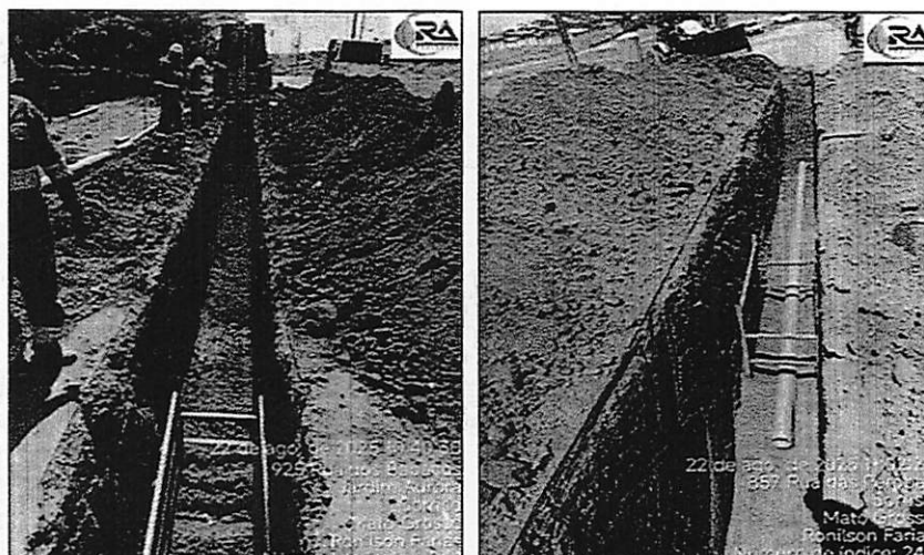
Figura 19. Assentamento da rede coletora
