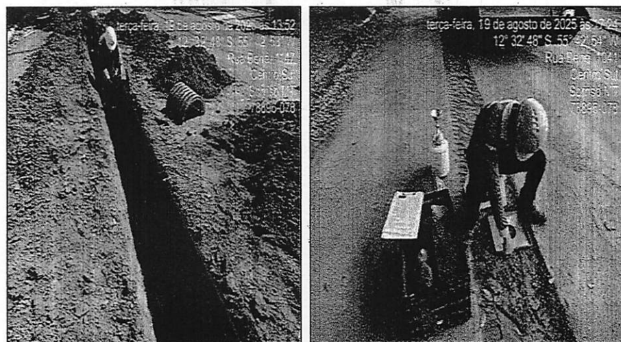
Figura 6. Escavação para implantação da linha de recalque e análise da compactação do solo
