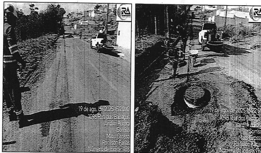
Figura 9. Implantação do poço de visita
