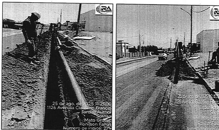
Figura 27. Escavação e assentamento de tubos
