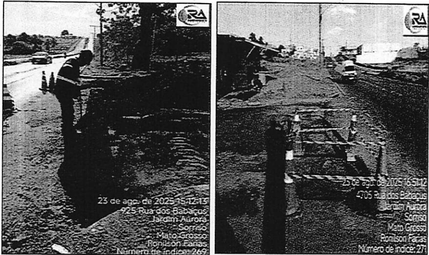
Figura 24. Implantação de poço de visita
