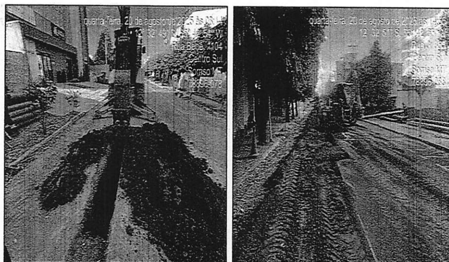
Figura 10. Assentamento de tubos e recomposição do solo
