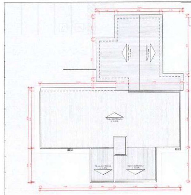
4 PLANTA DE COBERTURA - FINAL 1:125
