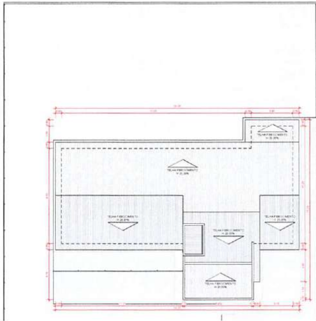
1 PLANTA DE COBERTURA - EXISTENTE 1:125
