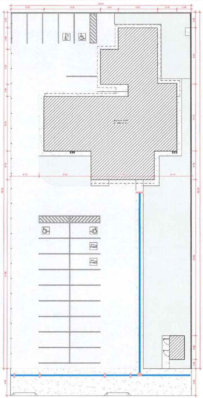
1 PLANTA DE IMPLANTAÇÃO 1 : 175
