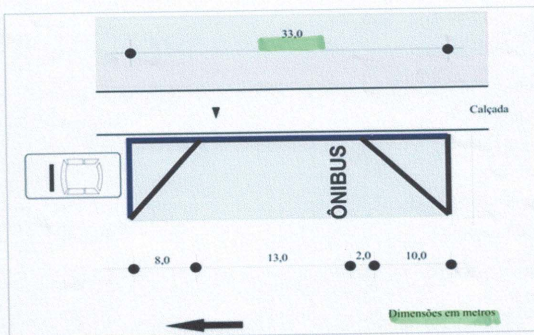
Figura 01 – Dimensões ideais dos pontos de parada para ônibus com 12 m de comprimento – FONTE: Coca¹
